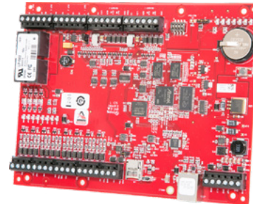
MRC-LP1502
